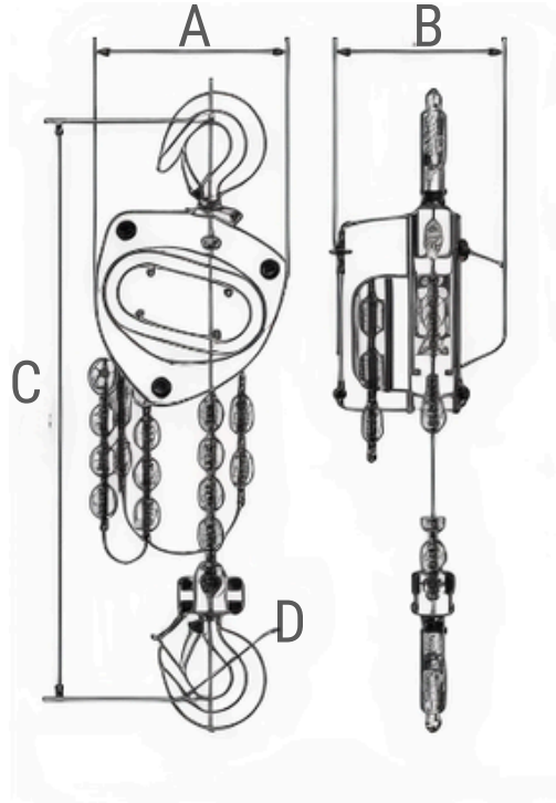
TECLE CADENA 500 Kg
